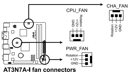
AT3N7A-I fan connectors
